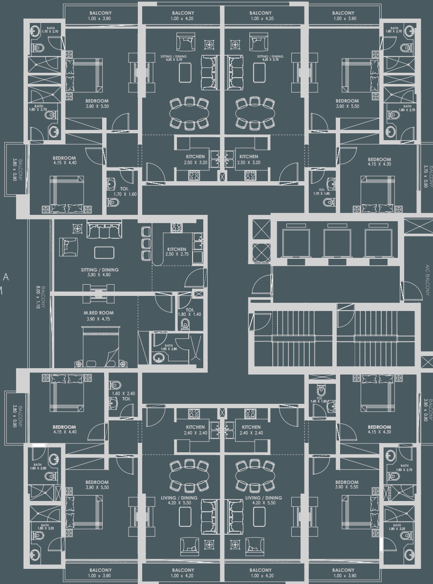
FLAT - 4: 2BR - TYPE A1 AREA = 111.68 SQM
